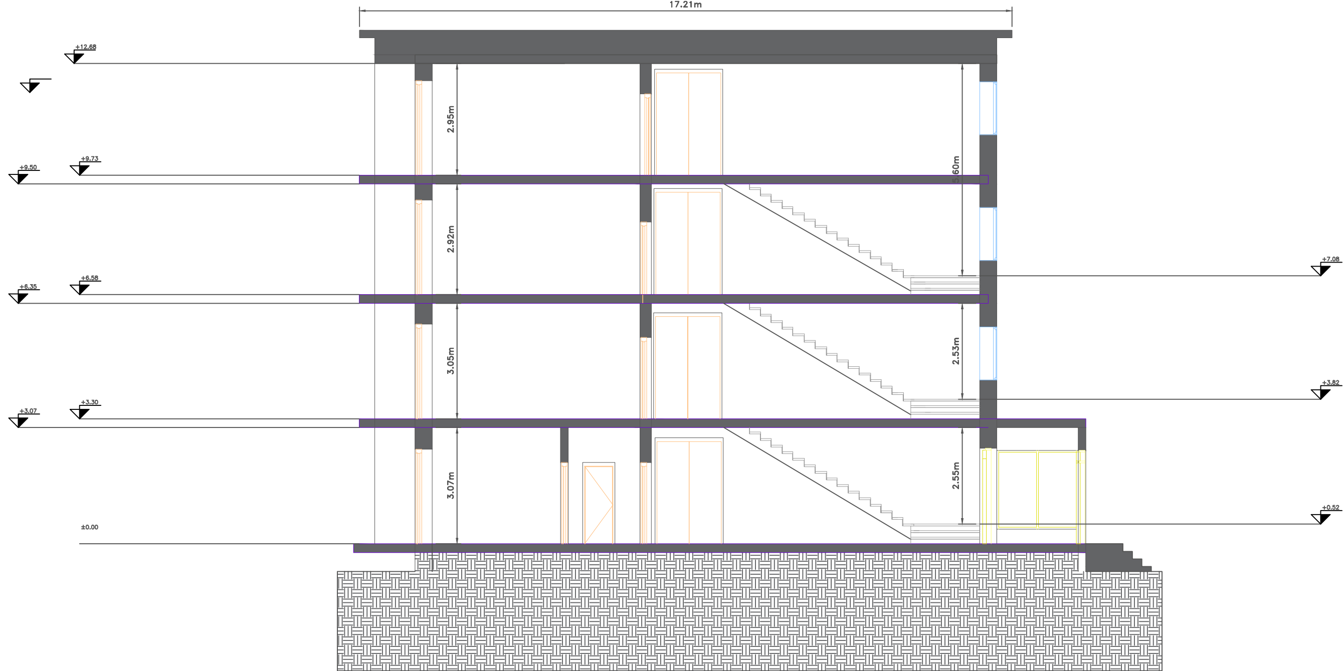
Sectiune 3-3
