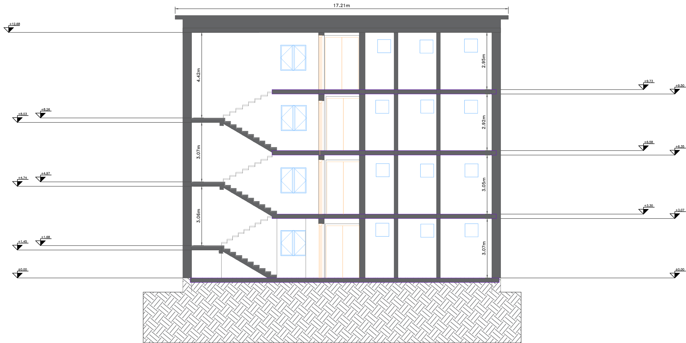
Sectiune 2-2
